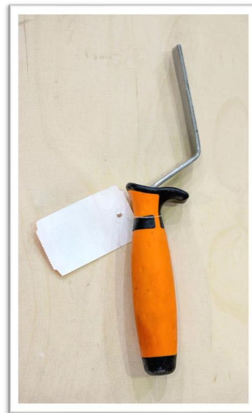
Pystysaumarauta
